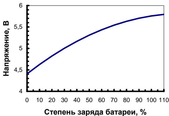
Рисунок 5.4 Заряд аккумулятора
